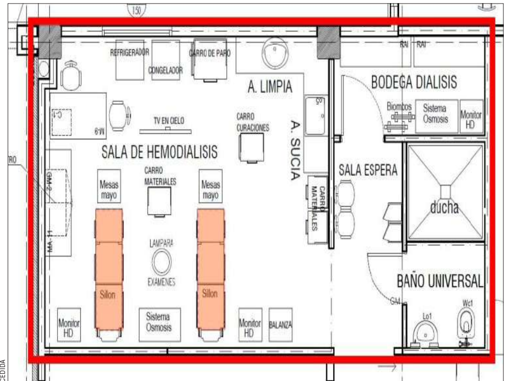
Plano de cómo estará distribuida la Unidad de Diálisis.
