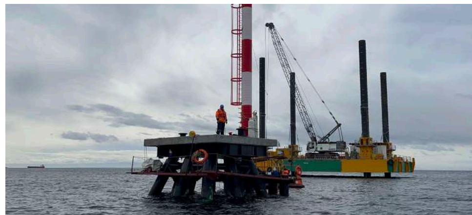
El poste de amarre, junto al nuevo dolphin, permitirán la llegada de embarcaciones sobre 300 metros de eslora.
